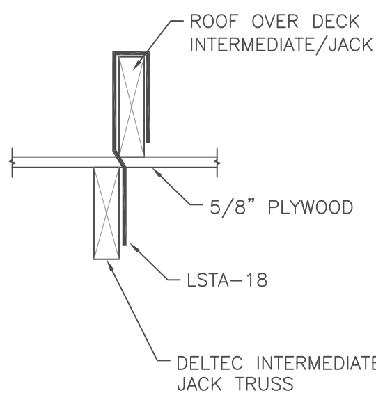
SECTION 9-H SCALE: 1-1/2"=1'-0"
